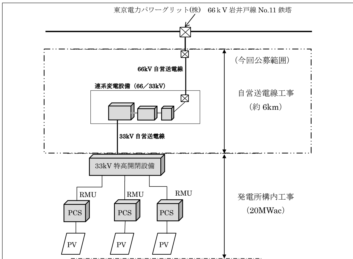
図 1.1 公募範囲概要図
